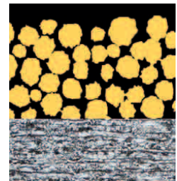
Mikroschliffbild AMV®-K
